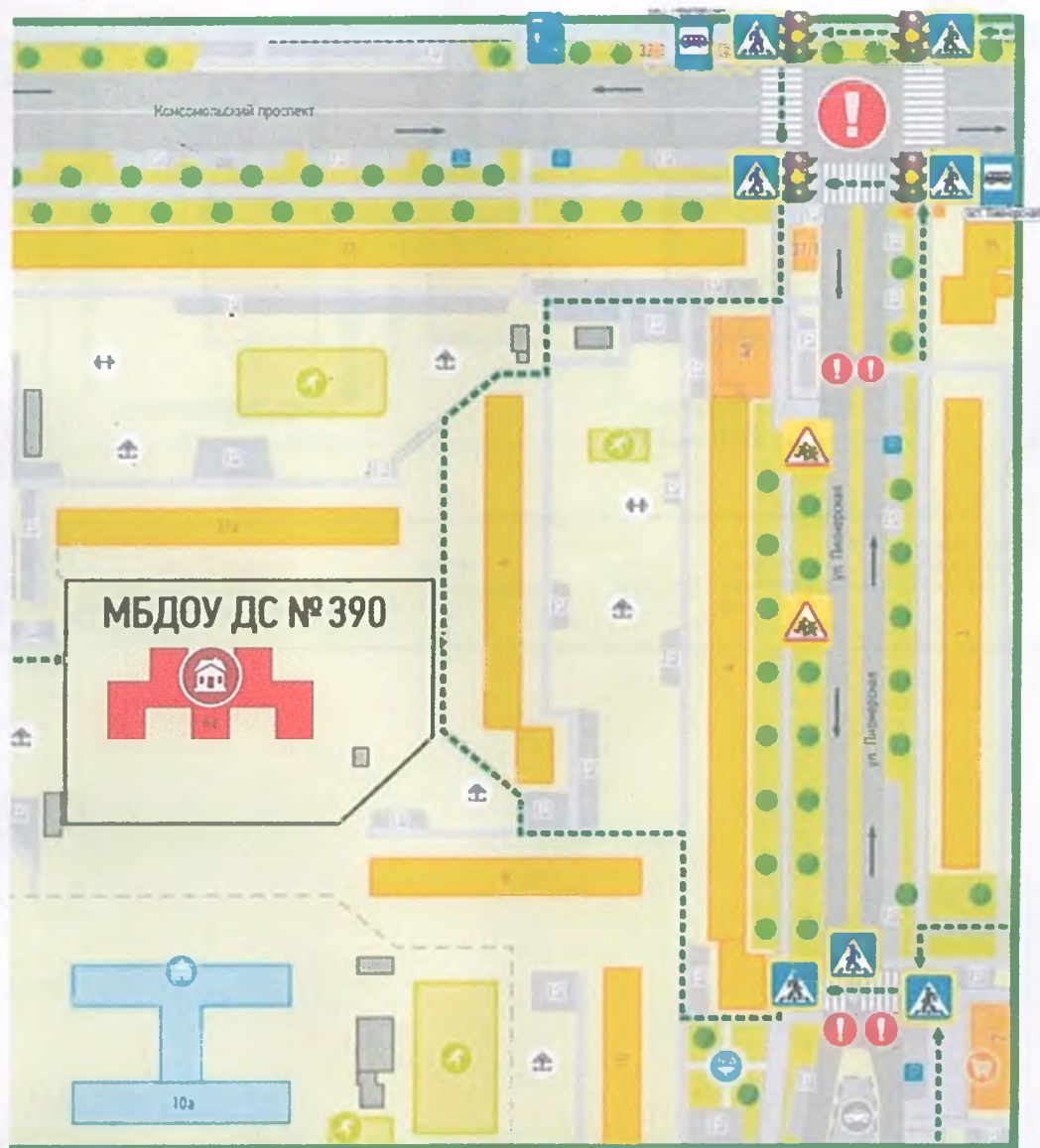
Схема 2. Организация дорожного движения в непосредственной близости от образовательного учреждения с размещением соответствующих технических средств, маршруты движения детей и расположение парковочных мест
